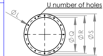
Optional Inlet Flange
